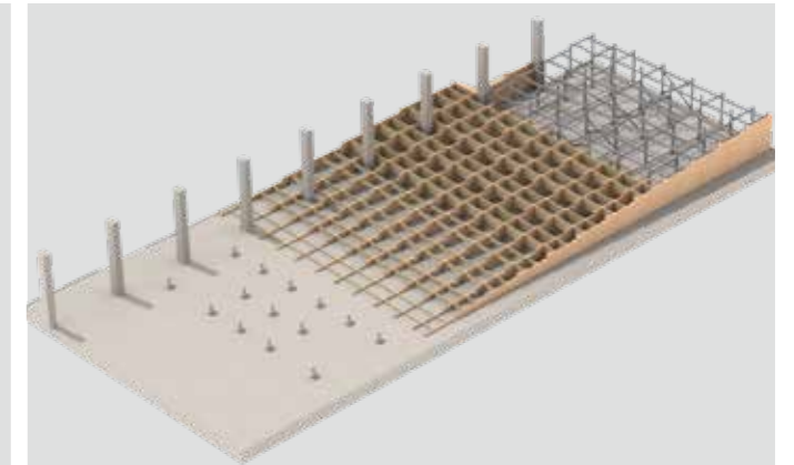
2 CAD – Unterkonstruktion
